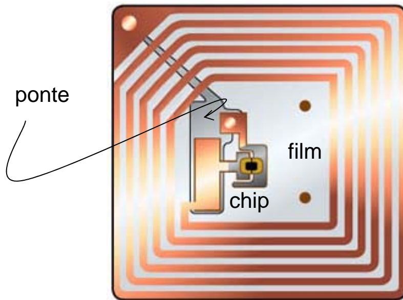
Avvolgimento (coil)
